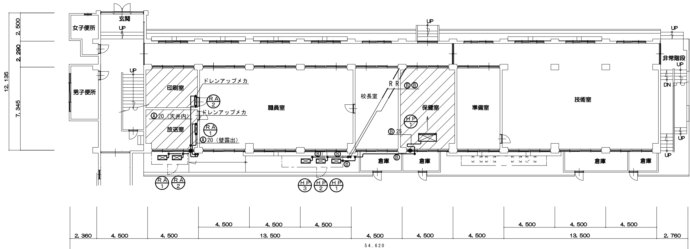
本館1階平面図 S = 1/200
