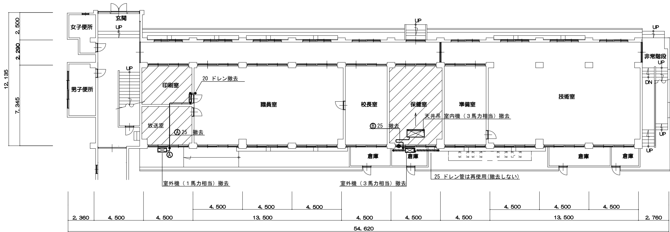
本館1階平面図 S = 1 / 2 0 0
