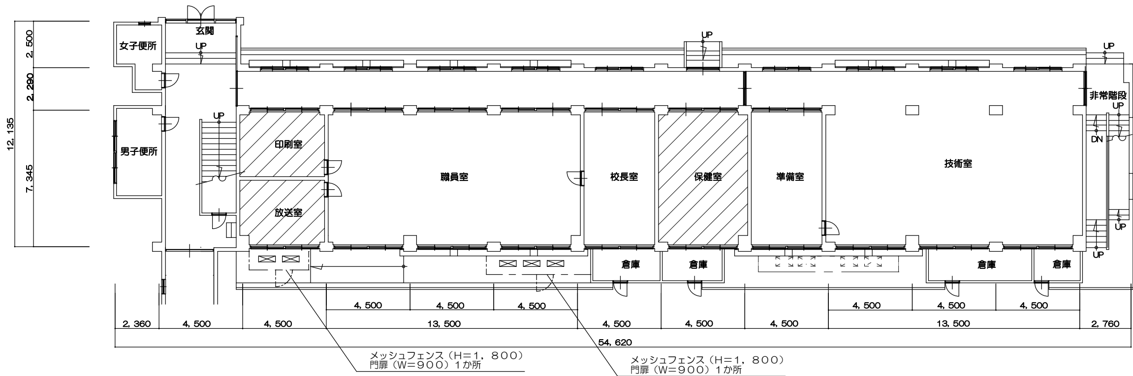
本館1階平面図 S = 1 / 2 0 0
