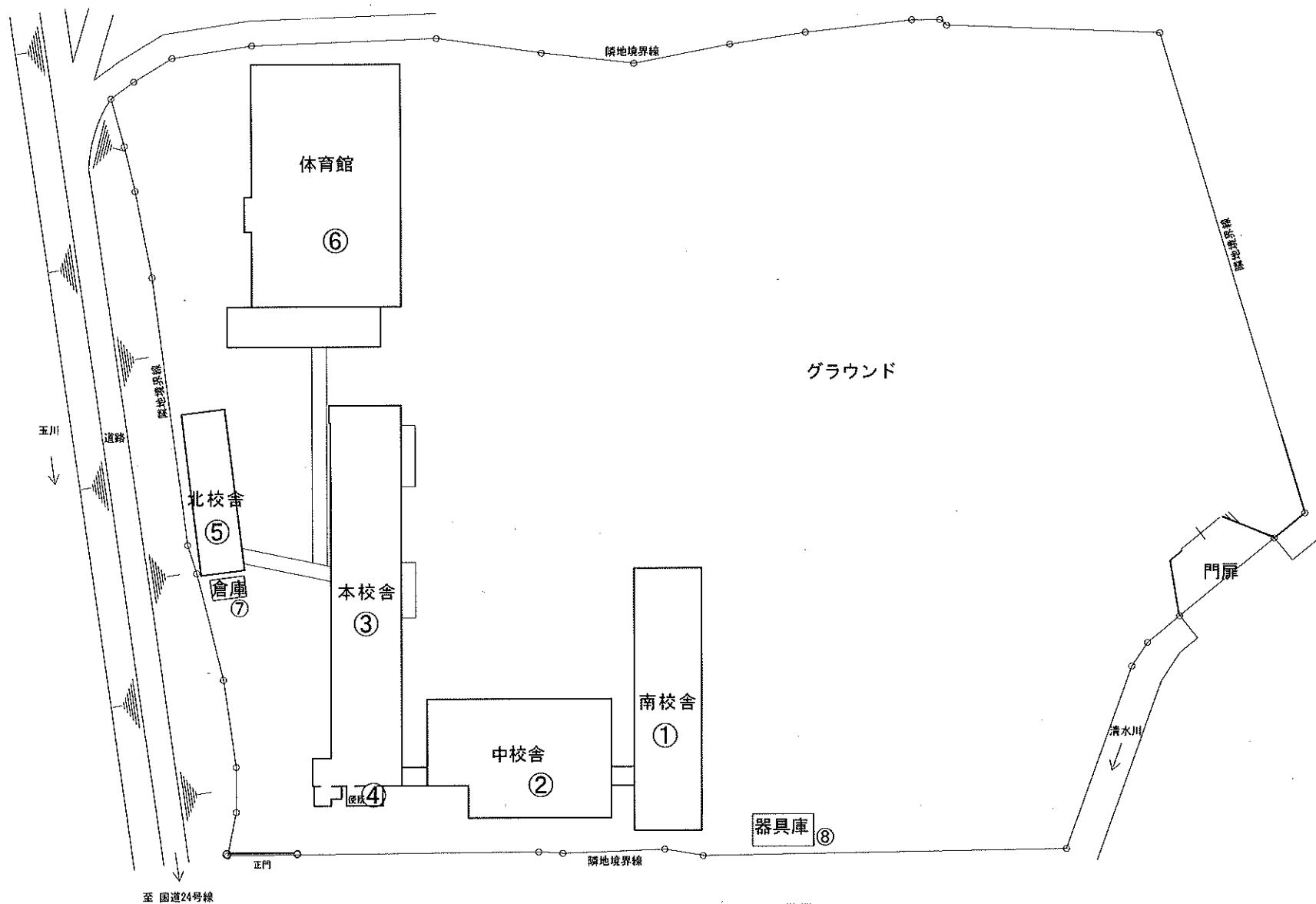
泉ヶ丘中学校 配置図
